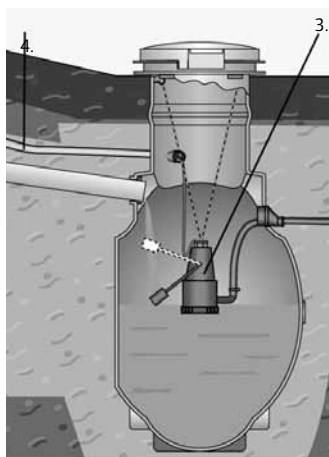
Uppopumppu asennettuna pumppukaivoon.
