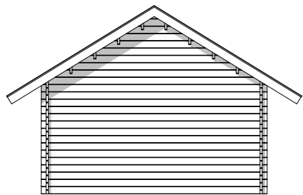
Fasad 1:100
