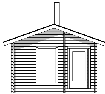
Fasad 1:100
