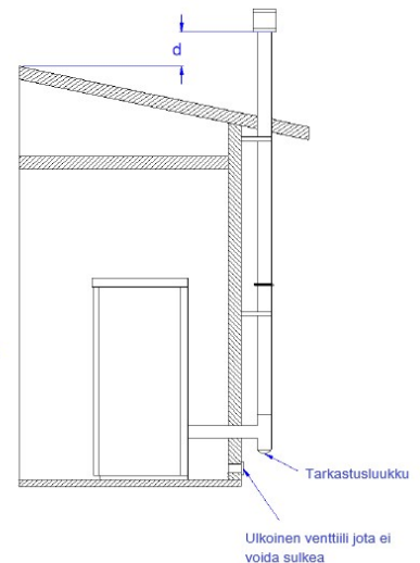
ULKOINEN SAVUPIIPPU:
